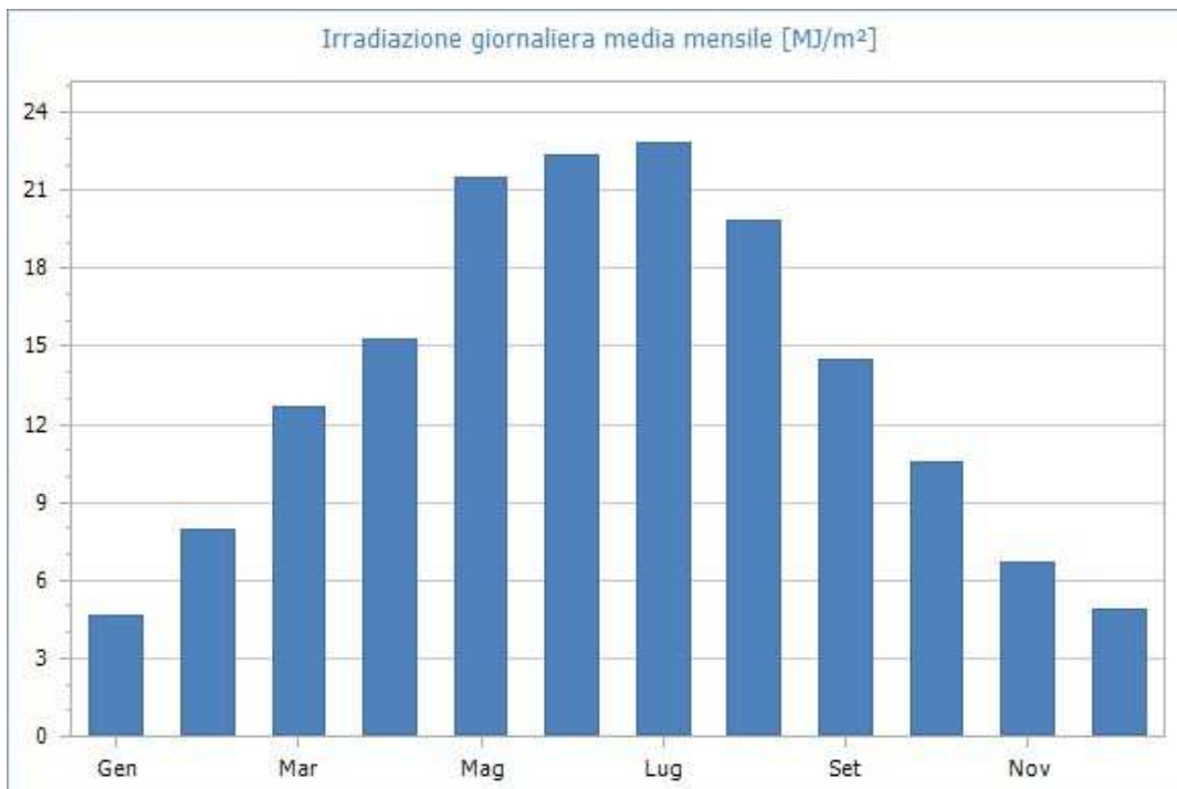
Fig. 1: Irradiazione giornaliera media mensile sul piano orizzontale [MJ/m²]- Fonte dati: UNI 10349:2016 - Stazione di rilevazione: Nuoro
