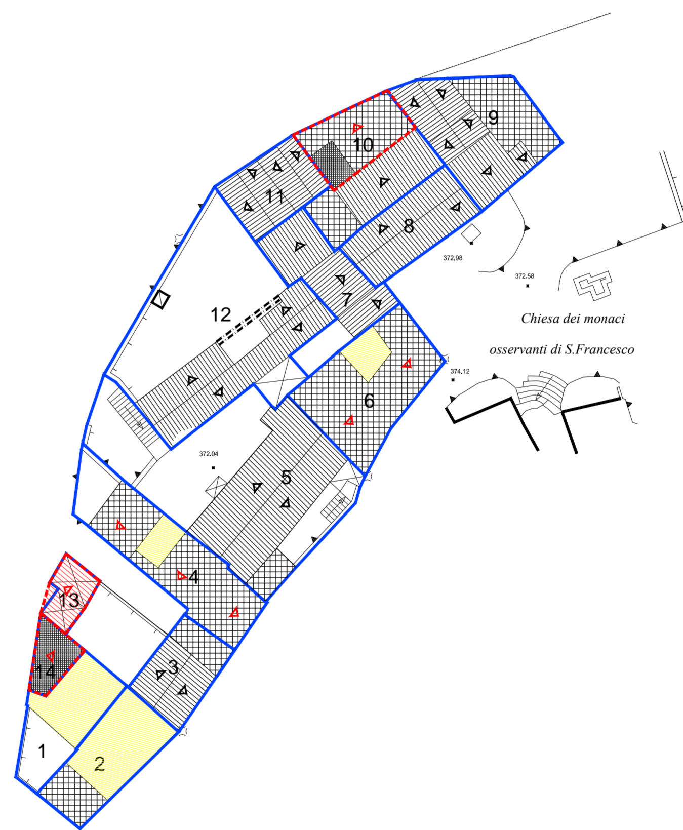
PLANIMETRIA QUINTO LIVELLO
